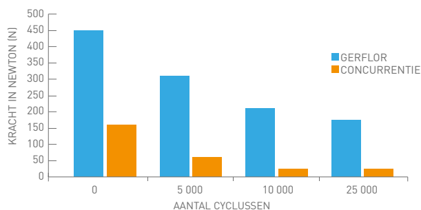
MECHANISCHE EIGENSCHAPPEN (Modulus* N) NF T 54-103
